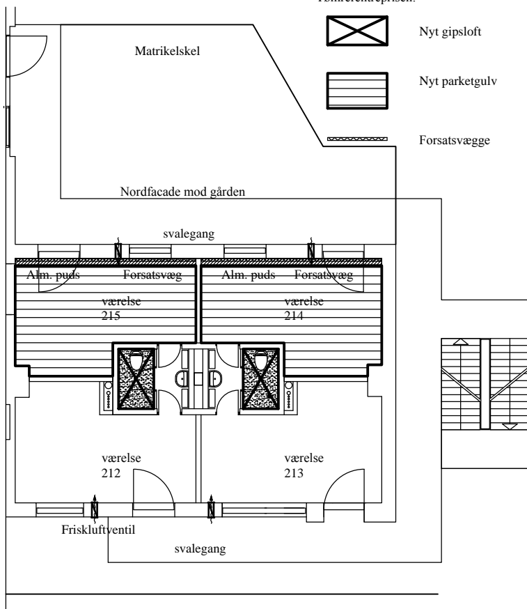
Værelsesudsnit 1.sal
